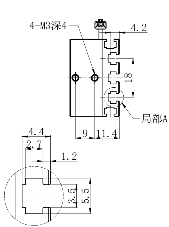
局部A 比例3:1 M3螺母凹槽, 安装用
