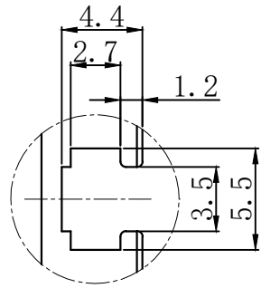
局部A 比例3:1 M3螺母凹槽，安装用
